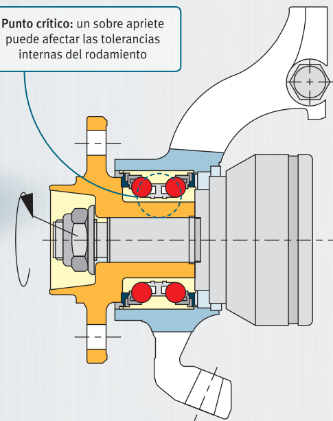
Tuerca de seguridad en un ensamble convencional
