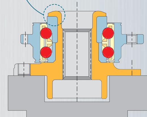
Diseño Orbital FAG
